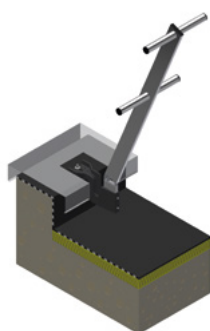
Support Eco-Line T17 incliné Fixation sous couvertine (acrotère non isolé)
