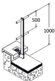
Eco-Line sous couverture (acrotère non isolé)
