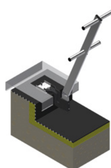
Support Eco-Line T17 Fixation sous couvertine (acrotère isolé)
