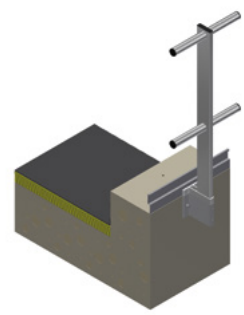
Support Eco-Line T17 Fixation en applique (extérieur acrotère)
