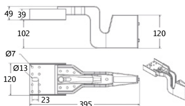
Platine Z rallongée
