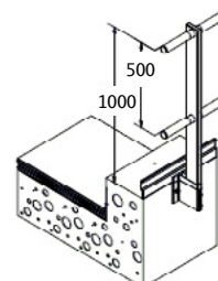
Eco-Line en applique (extérieur acrotère)
