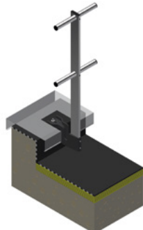
Support Eco-Line Fixation sous couvertine (acrotère non isolé)
