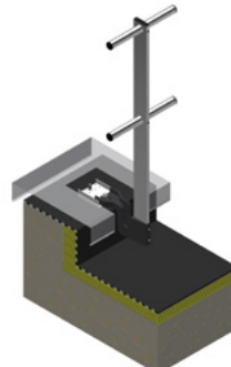
Support Eco-Line T17 Fixation sous couvertine (acrotère isolé)
