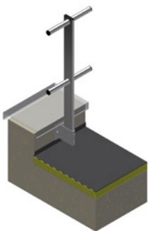
Support Eco-Line T17 Fixation en applique (intérieur acrotère)
