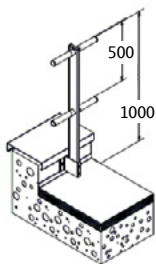
Eco-Line en applique
