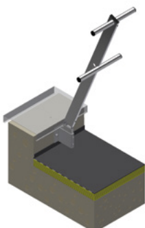
Support Eco-Line T17 incliné Fixation en applique (intérieur acrotère)
