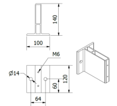
Platine applique extérieur
