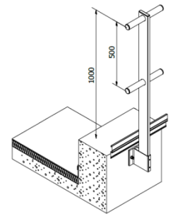
Eco-Line T17 en applique (extérieur acrotère)
