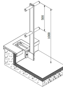
Eco-Line T17 sous couvertine (acrotère isolé)
