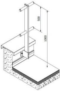
Eco-Line T17 en applique (intérieur acrotère)
