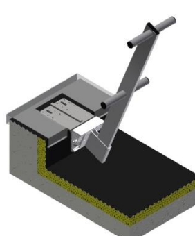
Support Eco-Line T17 incliné Fixation sous couverture (acrotère isolé)
