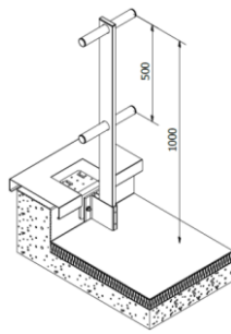
Eco-Line T17 sous couvertine (acrotère non isolé)
