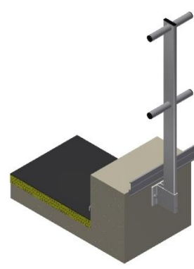
Support Eco-Line T17 Fixation en applique (extérieur acrotère)
