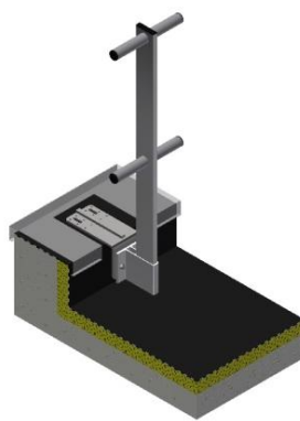
Support Eco-Line T17 Fixation sous couverture (acrotère isolé)
