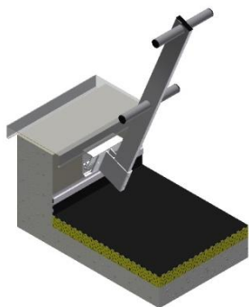
Support Eco-Line T17 incliné Fixation en applique (intérieur acrotère)
