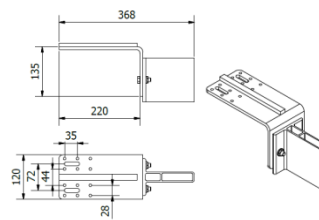
Platine Z rallongée
