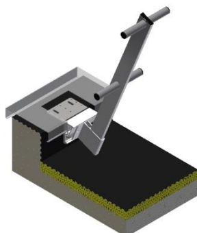
Support Eco-Line T17 incliné Fixation sous couverture (acrotère non isolé)
