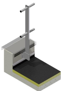
Support Eco-Line T17 Fixation en applique (intérieur acrotère)
