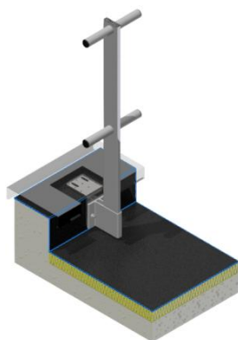
Support Eco-Line T17 Fixation sous couverture (acrotère non isolé)
