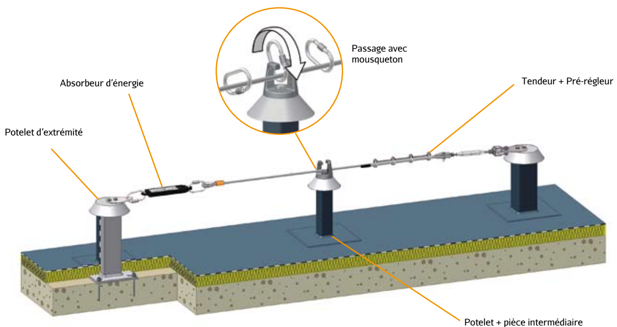
Ligne de vie ECOVIE scellée sur dalle béton
