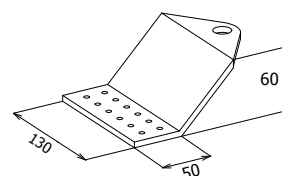
Ancrage d'extrémité Fixation parallèle au bac
