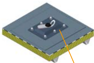
Fixation sur bac étanché et membrane PVC par 2 chevilles à bascule. (Épaisseur mini du bac support d'étanchéité 0.63mm).
