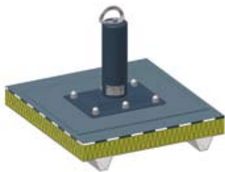
Fixation sur bac étanché et membrane PVC par 2 chevilles à bascule. (Épaisseur mini du bac support d'étanchéité 0,63mm).
