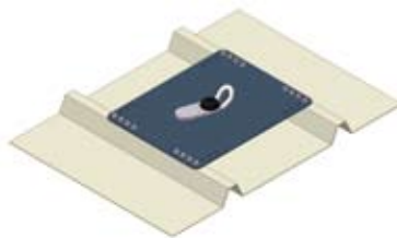
Fixation sur bac sec et panneaux sandwich par des vis autoperçantes munies de rondelles d'étanchéité. (Épaisseur mini du bac 0,75mm).
