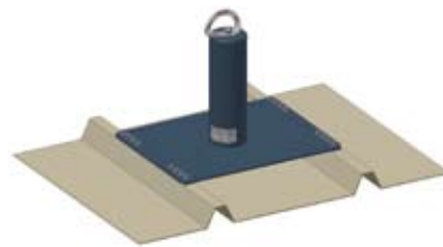
Fixation sur bac sec et panneaux sandwich par des vis autoperceuses munies de rondelles d'étanchéité. (Épaisseur mini du bac 0,75mm).
