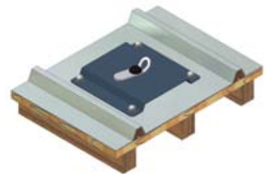
Fixation sur zinc-volige par 4 chevilles à bascule. (Épaisseur mini de la volige 12mm).
