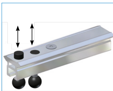
Butée d'extrémité mobile, qui permet l'entrée/sortie du chariot sur le rail en actionnant les plots mobiles
