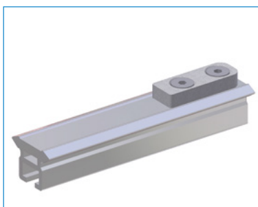
Butée d'extrémité fixe, montée sur le rail pour stopper le déplacement du chariot à l'extrémité du dispositif
